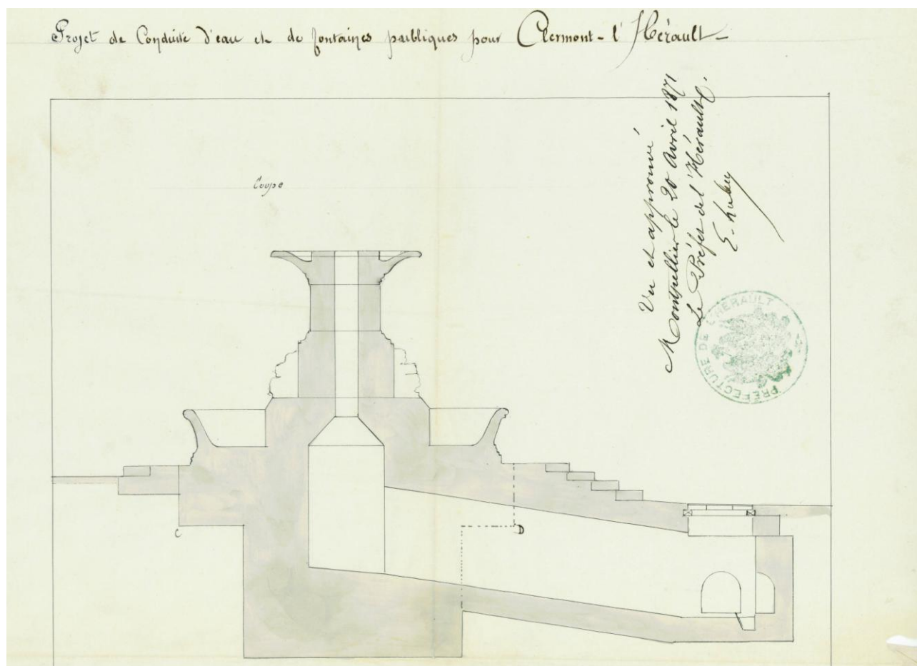
Projet de conduite d'eau et de fontaines publiques (1871) 3N1
