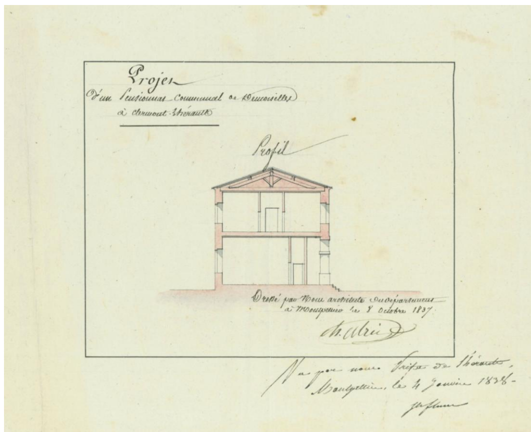
Projet d'un pensionnat communal de demoiselles (1837)
