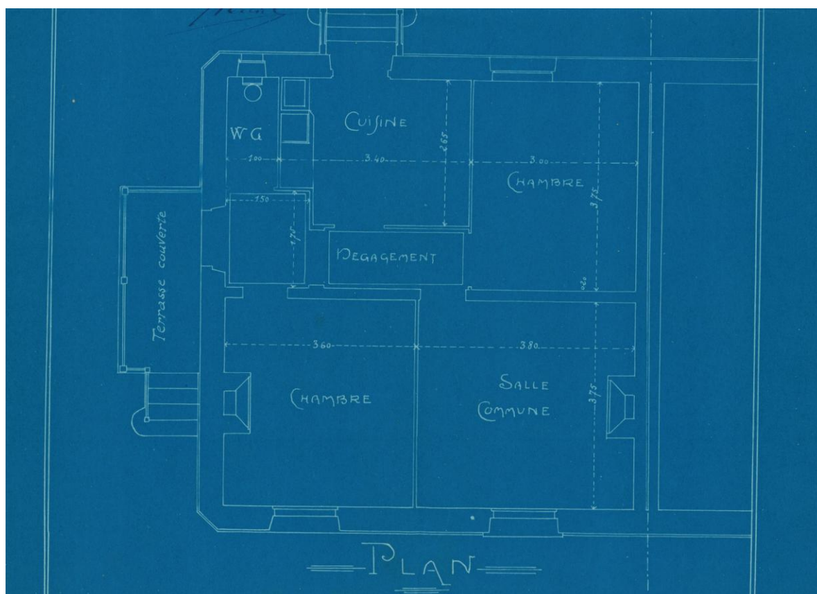
Plans d'habitations bon marché (1924) T41
